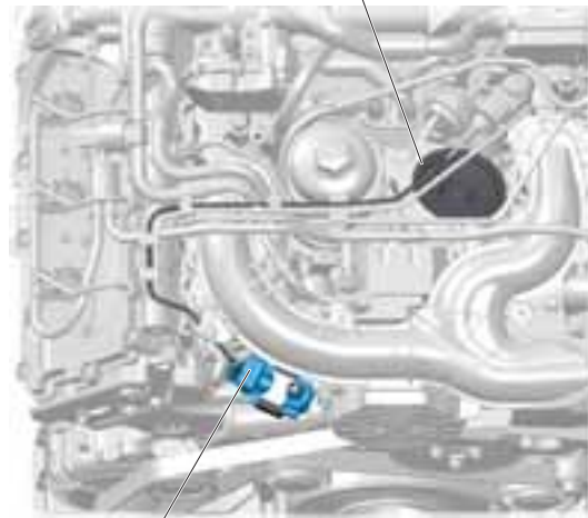
Abgasrückführungsventil N18
