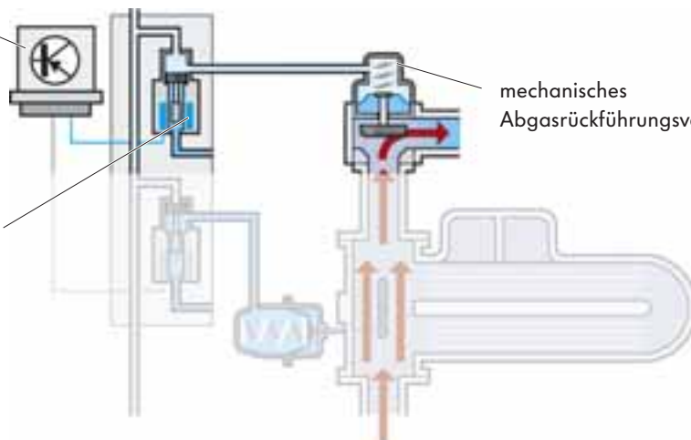
Abgasrück- führungsventil N18
